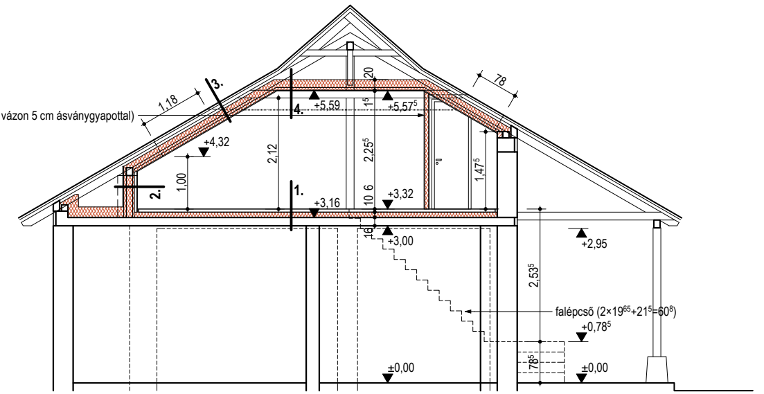
METSZET m=1:100
